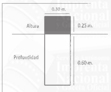
Diseño de Monumentación
