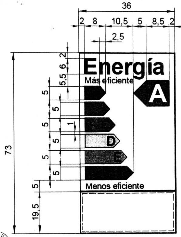
Figura N° 1. Dimensiones de la etiqueta en milímetros (mm)
