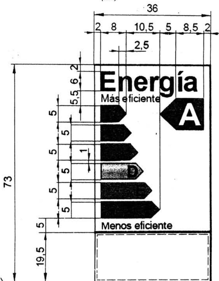
Figura N° 1. Dimensiones de la etiqueta en milímetros (mm)
