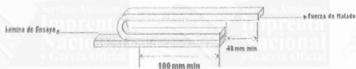
Figura 6. Fuerza de halado a 180° de la etiqueta adhesiva
