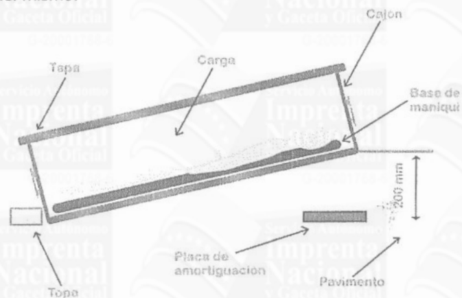
Figura 6. Determinación de la Resistencia a Impactos
