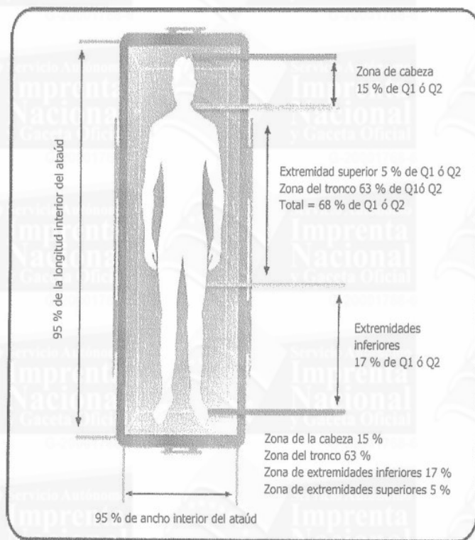
Figura 2. Distribución de las cargas
