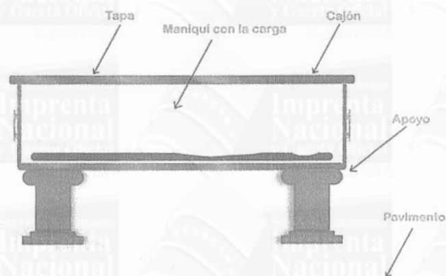
Figura 5. Determinación de la Resistencia de la Estructura del Ataúd
